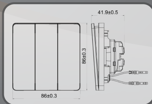
■ 三切開關產品尺寸(mm)
